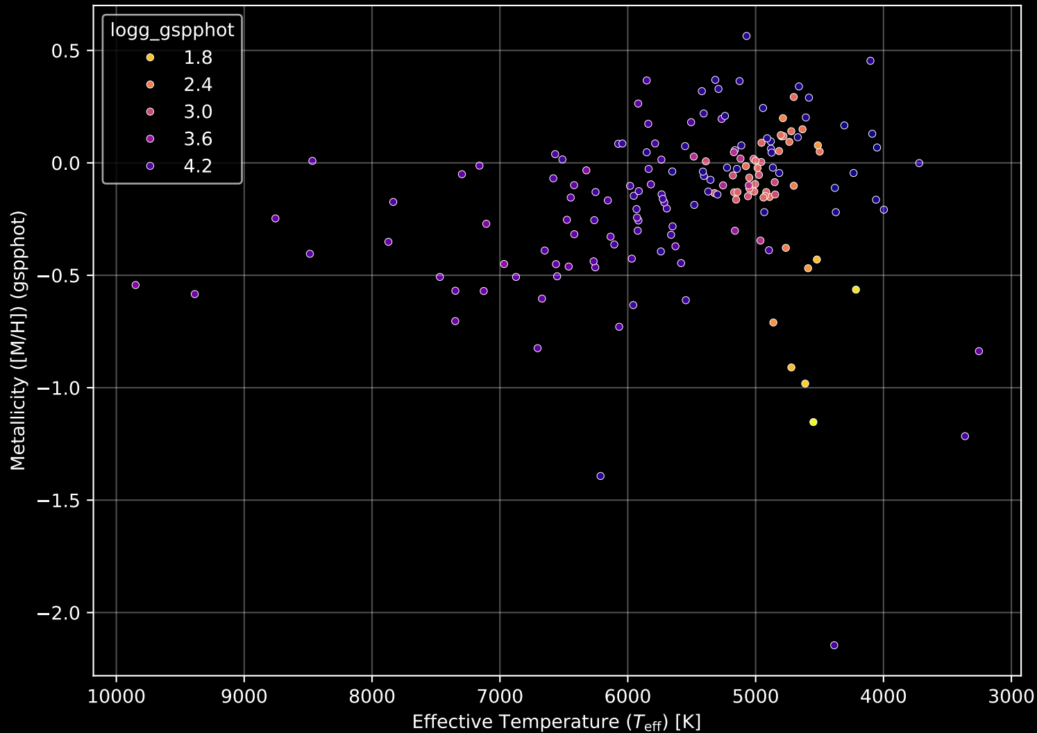
APOGEE DR17 Field: [CVZTILE_103+22_btx] Stellar Population Parameters (n= 166)
